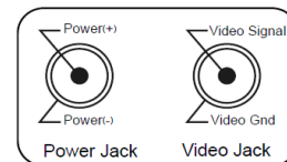
Connessione Cavi
